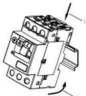
Рис. 3. Установка автоматического выключателя ВА-431 на дин-рейку.
