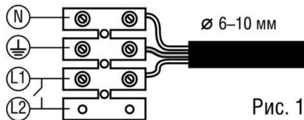
Схема подключения БАП в светильнике NLP-S2-A
