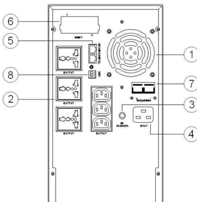
Корпус Tower. Задняя панель ИБП 3 кВА
