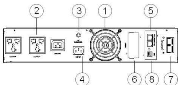
Корпус Rack Tower. Задняя панель ИБП 1 кВА
