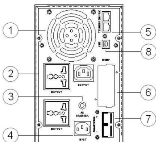
Корпус Tower. Задняя панель ИБП 1 – 2 кВА
