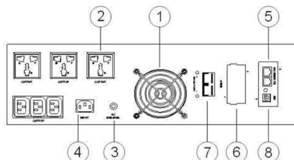
Корпус Rack Tower. Задняя панель ИБП 1.5 кВА – 3 кВА
