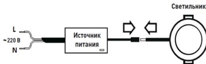
Рис.1. Подключение светильника к сети переменного тока 220В.
