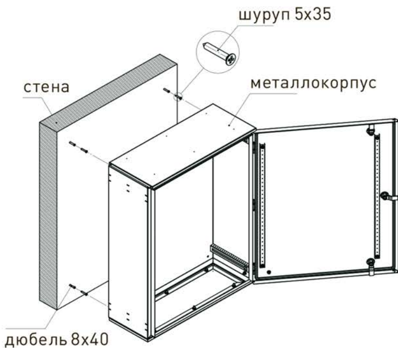
Рис. 1.1. Схема настенного монтажа.
