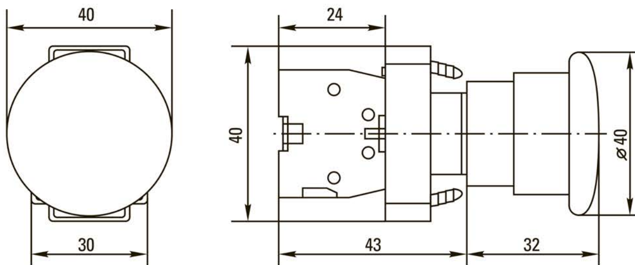
КНОПКИ BS542, BC42
