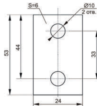
Рисунок 7в – Наконечник переходник для BA88-37M
