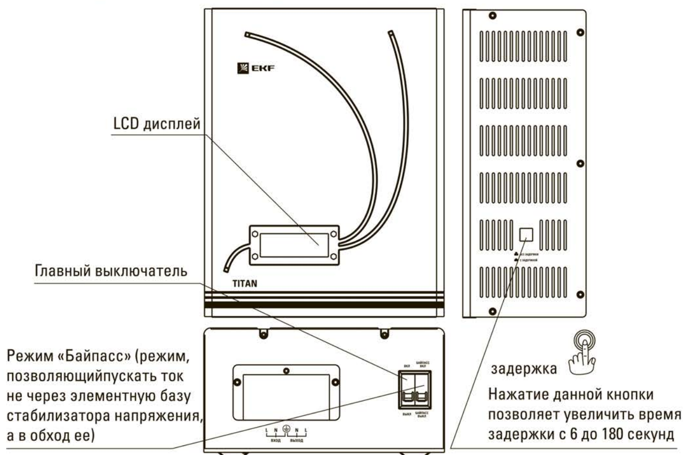
Рис. 2 Внешний вид стабилизатора W-8000/10000/12000
