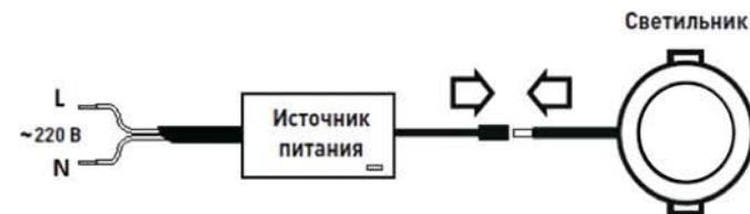
Рис.1. Подключение светильника к сети переменного тока 220В.
