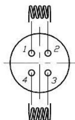
Схема соединения выводов в цоколе
