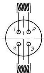
Схема соединения выводов в цоколе
