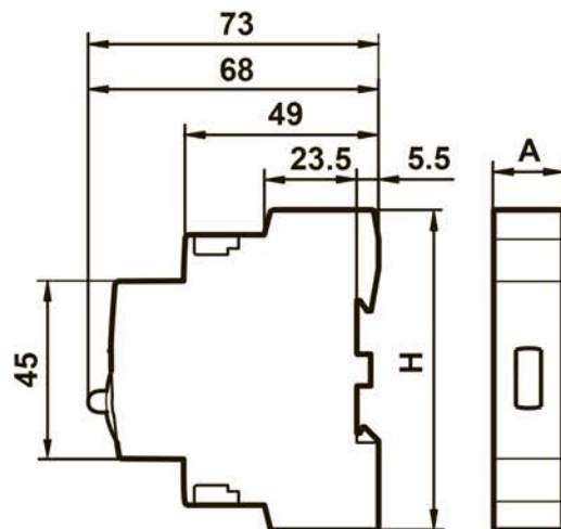
Рис. 1 - Габаритные размеры контакторов КМ РУ
