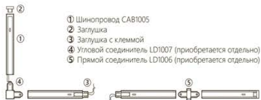
Угловое соединение
