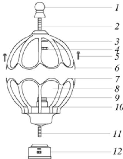
1 – балясина; 2 – резьбовое крепление; 3 – гровер; 4 – гайка; 5 – винты; 6 – верхняя крышка; 7 – нижняя крышка; 8 – рассеиватель; 9 – патрон; 10 – ламподержатель; 11 – резьбовое крепление; 12 – основание.
