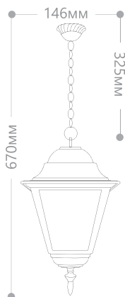
Схема НСУ-04-60-001
