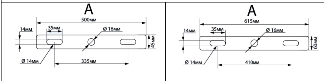
Схема монтажа основания:
