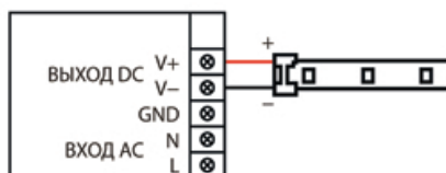
Схема подключения
