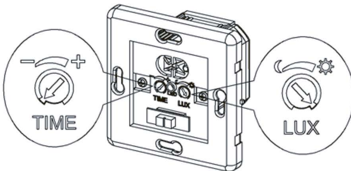
Рис.3. Начальные установки регуляторов во время настройки датчика.
