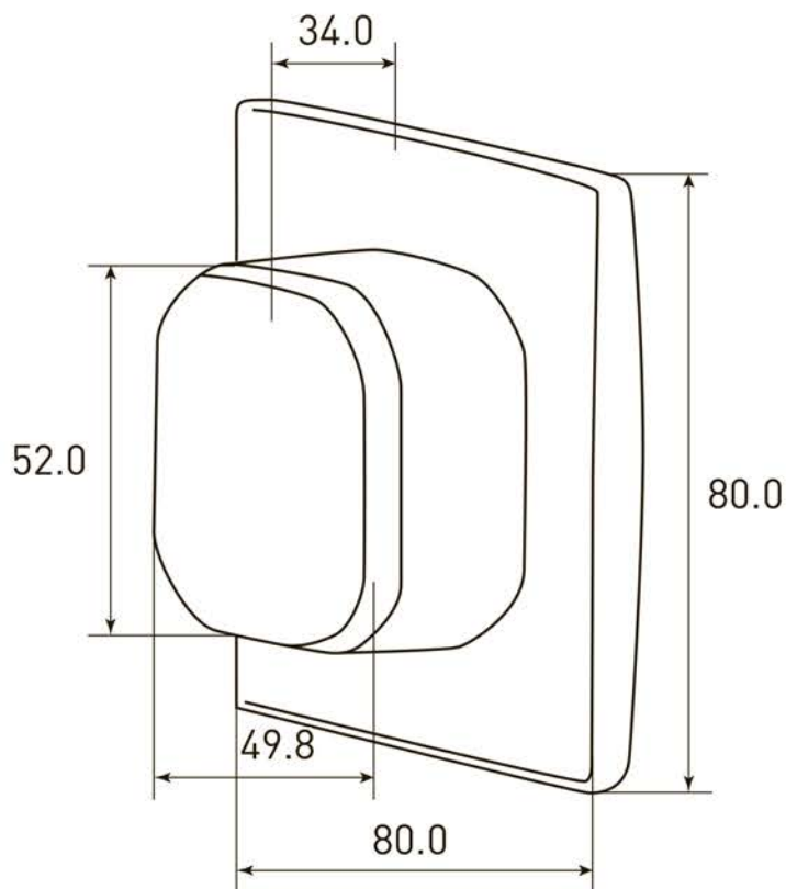
Рис.2. Габаритные размеры датчика движения.
