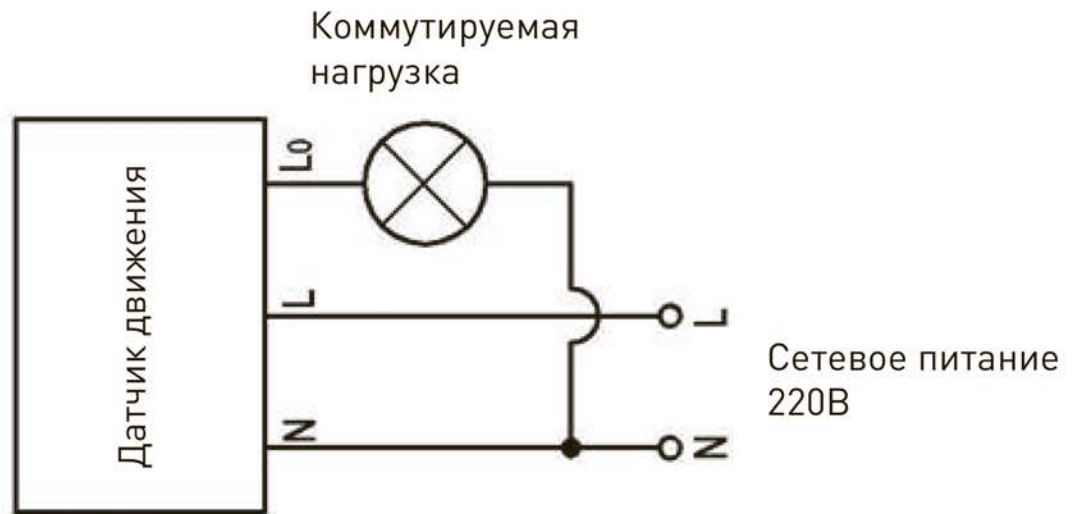
Рис.6. Подключение датчика движения.
