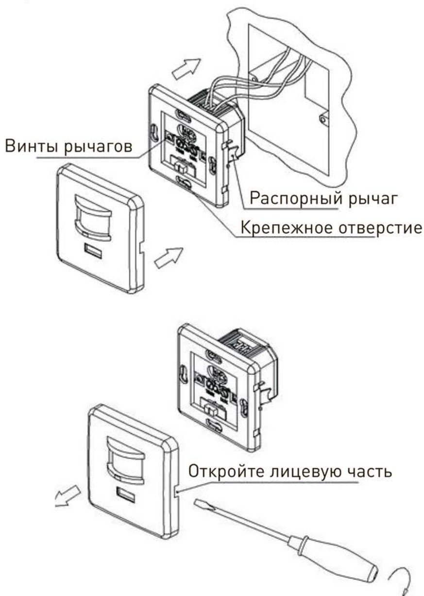
Рис.5. Разборка и крепление корпуса.
