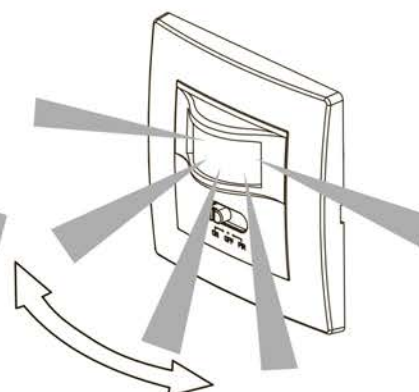
Рис.4. Диаграмма направленности зоны чувствительности.
