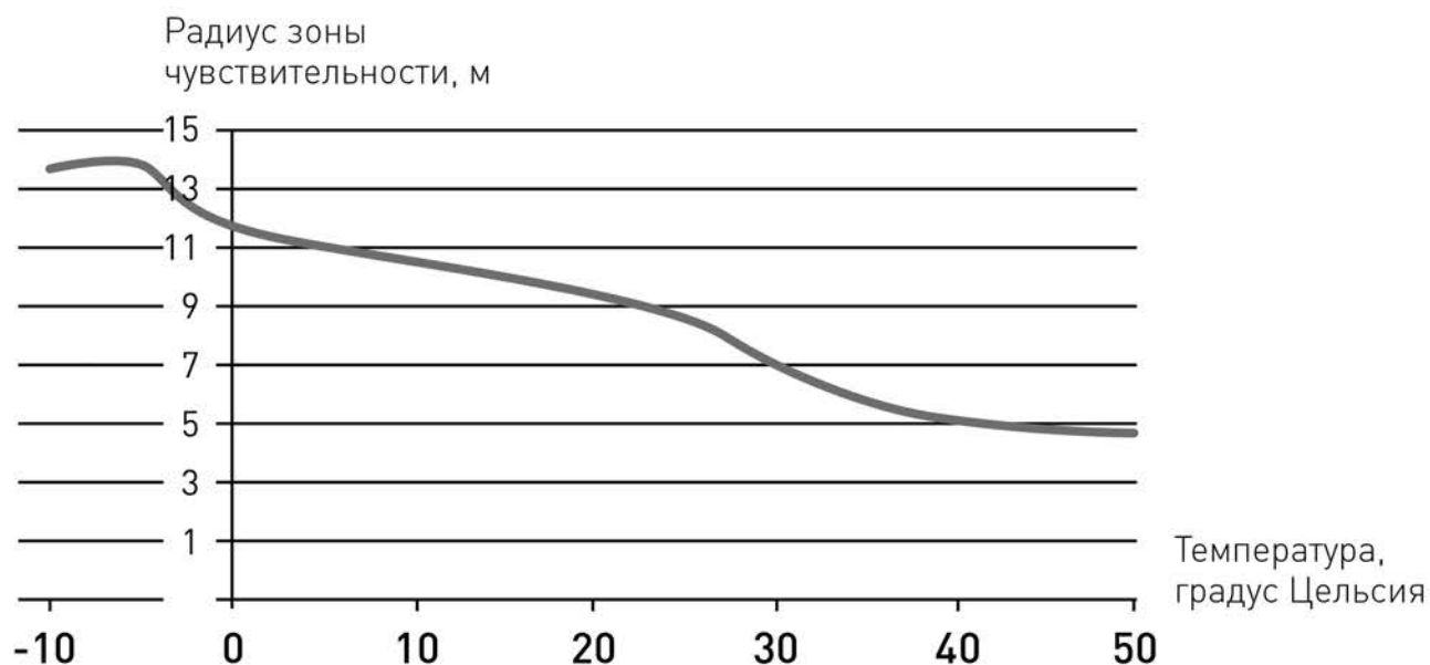
Рис.1. График зависимости радиуса зоны чувствительности от температуры.
