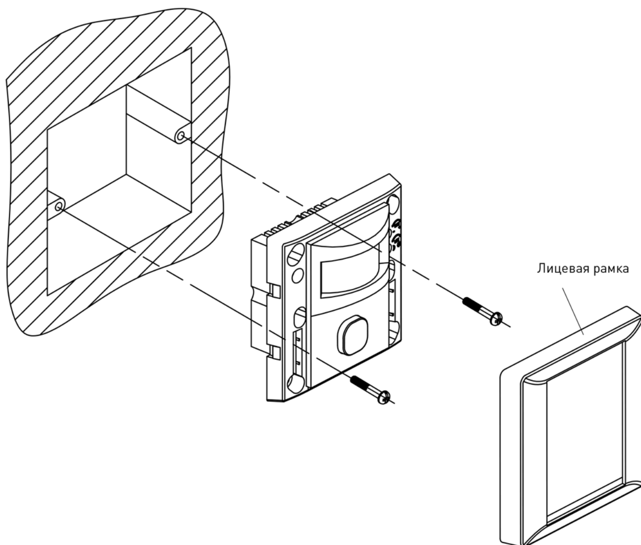
Рис.5. Разборка и крепление корпуса.
