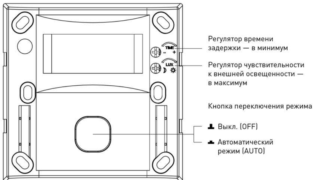
Рис.3. Начальные установки регуляторов во время настройки датчика.
