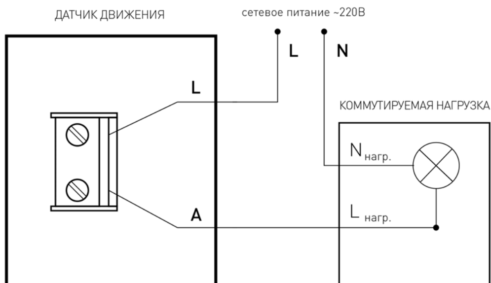
Рис.6. Подключение датчика движения.
