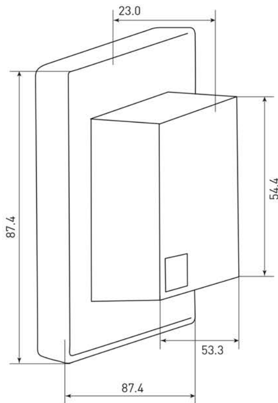
Рис.2. Габаритные размеры датчика движения.
