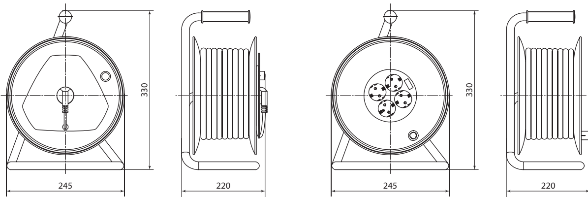
Удлинитель силовой со штепсельным гнездом УК10-001, УК6-001, УК310-001, УК316-001
