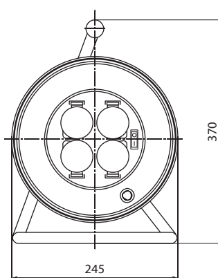
Удлинитель силовой с крышкой UX316-004, 4 места
