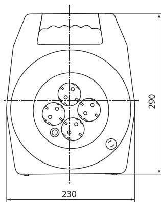
Удлинитель силовой в корпусе УК10-004, УК316-004, 4 места, 20 м
