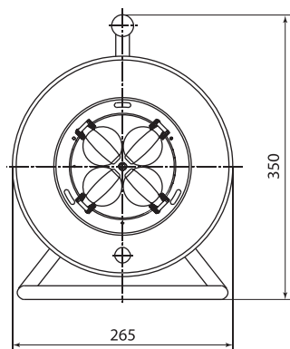
Удлинитель силовой с крышкой УК316-004, 4 места
