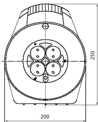
Удлинитель силовой в корпусе УК10-004, УК316-004, 4 места, 10 м
