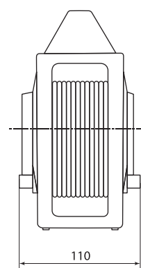
Удлинитель силовой в корпусе УК10-004, УК316-004, 4 места, 20 м
