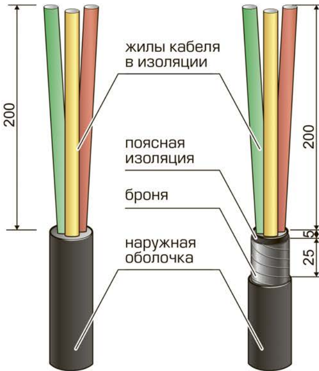
Кабель без брони
