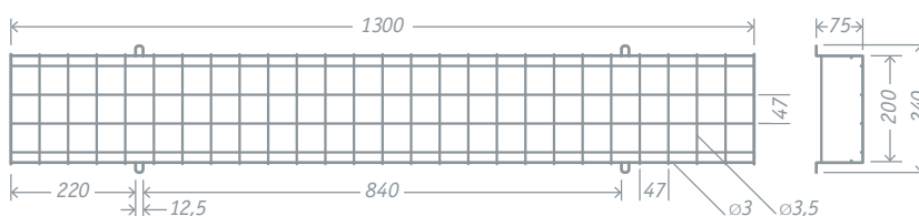
Размеры, мм
