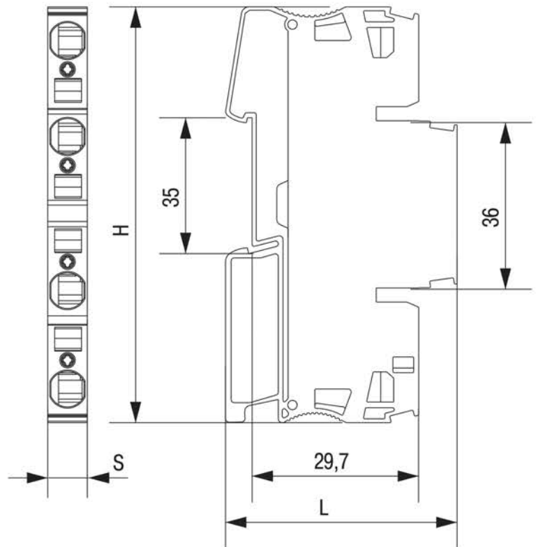
d) КПИ 4В-XX-2L
