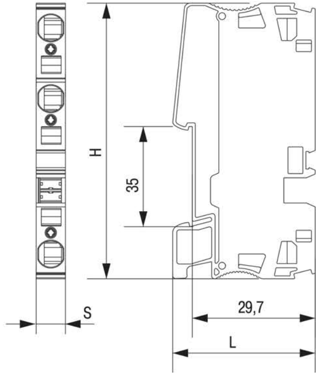
b) КПИ 3В-XX, КПИ 3В-XX-PEN
