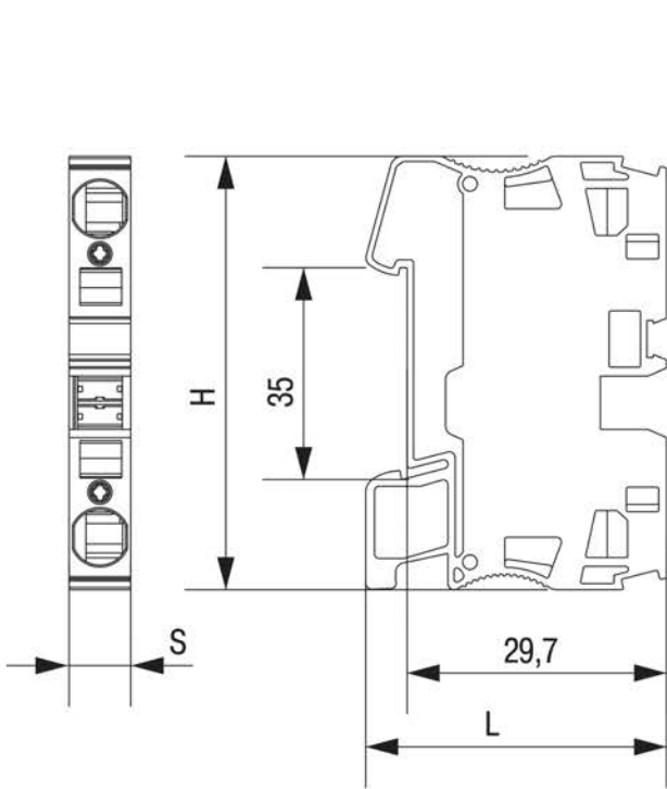
a) КПИ 2В-XX, КПИ 2В-XX-PEN
