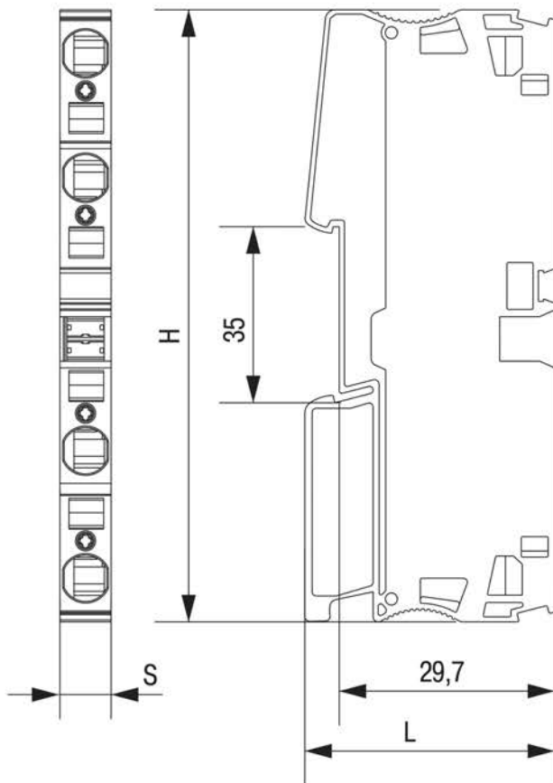
c) КПИ 4В-XX, КПИ 4В-XX-PEN
