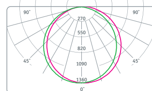
DPO-02-36-4K-IP20-LED
