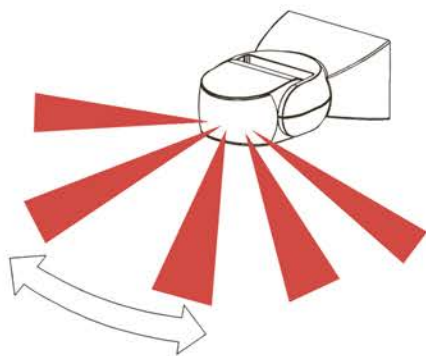
Высокая чувствительность при движении поперек зоны детектирования
