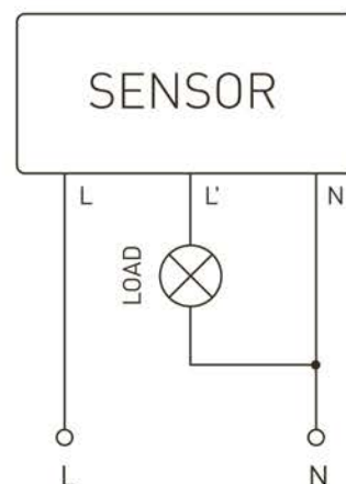
Рисунок 3. Схема подключения.
