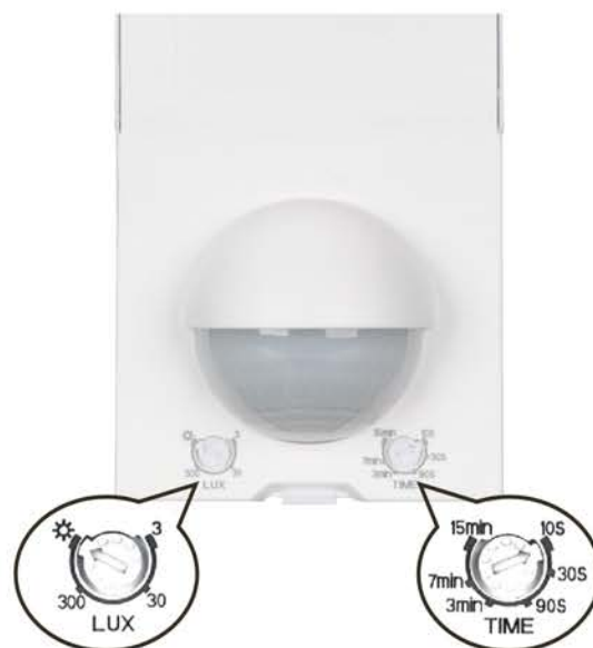
Рисунок 4. Регуляторы освещенности и времени задержки отключения.
