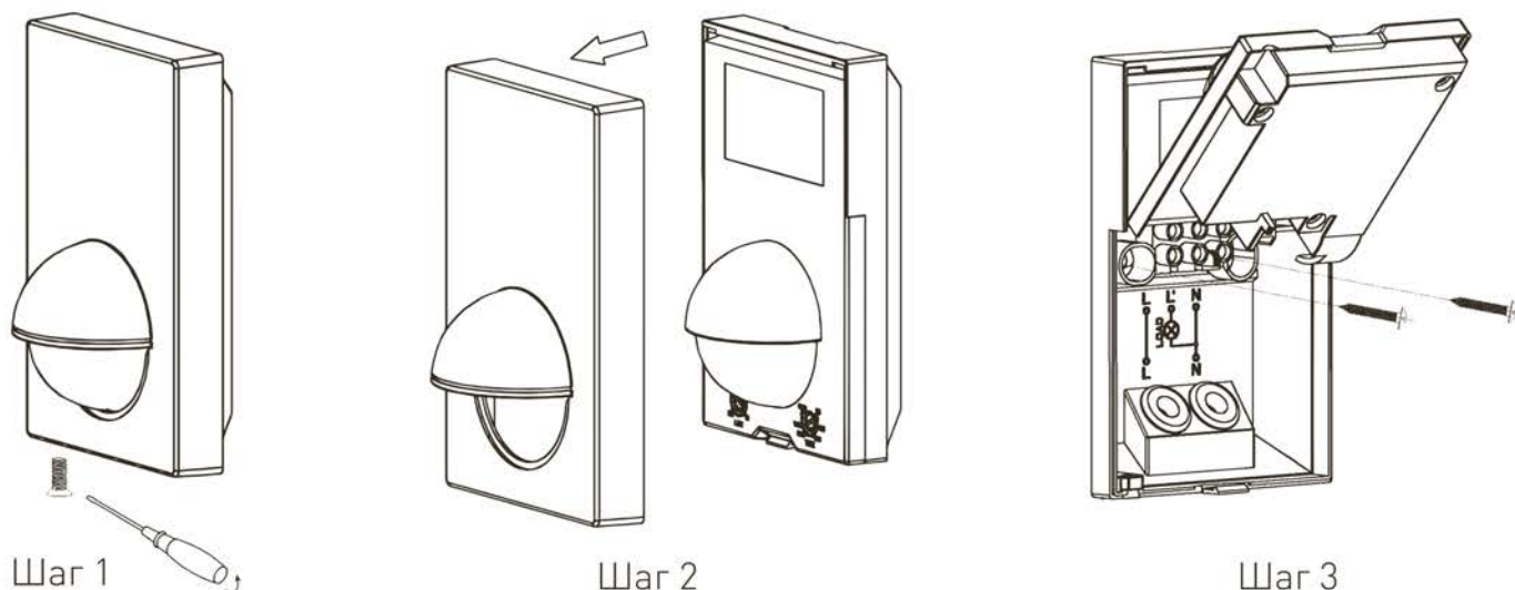
Рисунок 1. Этапы монтажа датчика.
