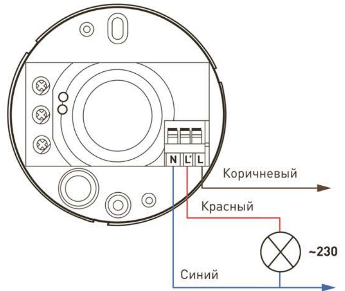
Рисунок 1. Схема подключения датчика движения.
