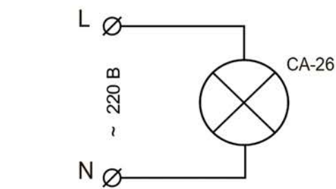
Рисунок 2 — Схема подключения основания СА-26 к питающей сети
