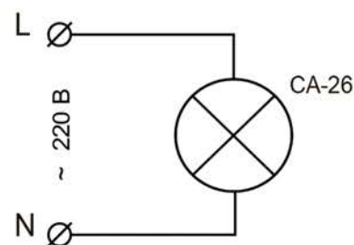
Рисунок 2 — Схема подключения основания СА-26 к питающей сети
