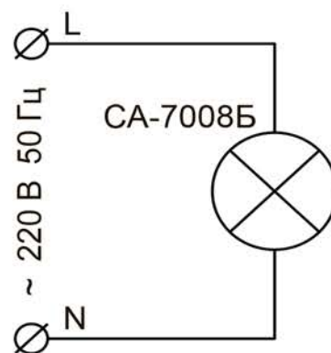
Рисунок 6 — Схема подключения светильника CA-7008Б
