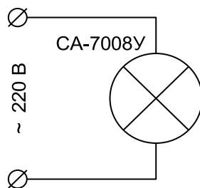
Рисунок 3 — Схема подключения светильника CA-7008Y
