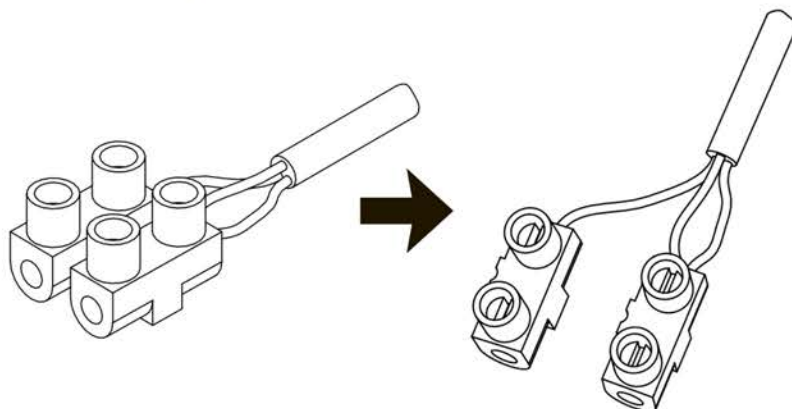
Рисунок 3 — Разделение секций клеммной колодки
