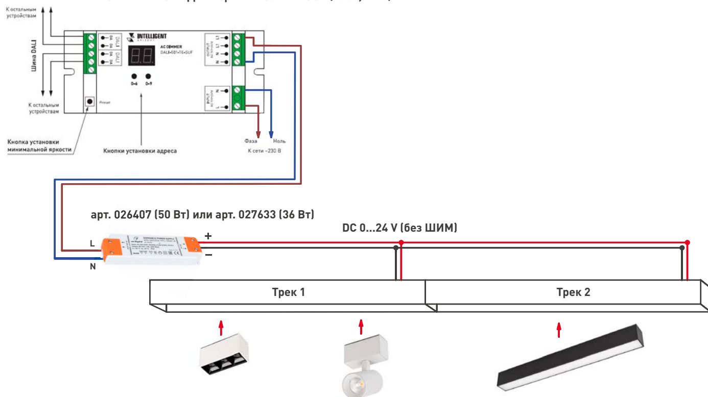
арт. 026403 INTELLIGENT ARLIGHT Диммер DALI-501-TE-SUF (230V, 2.2A)
