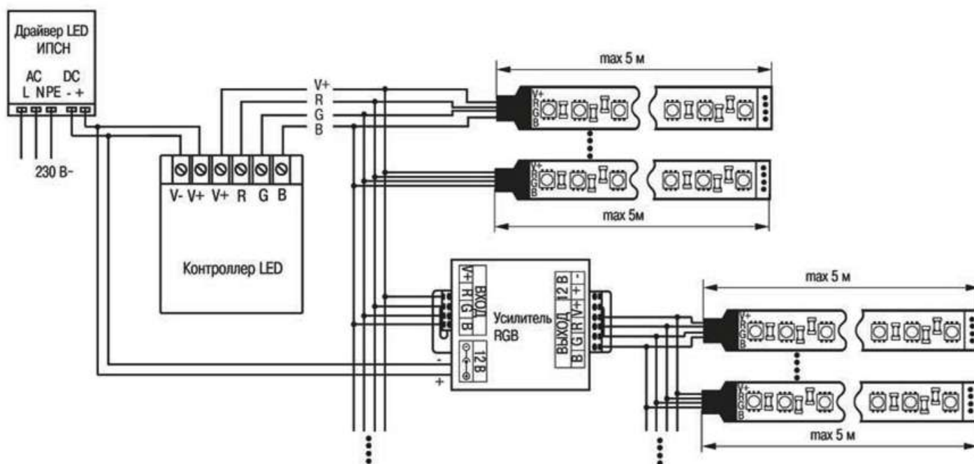
Рисунок 9 – Схема параллельного подключения RGB-усилителя
