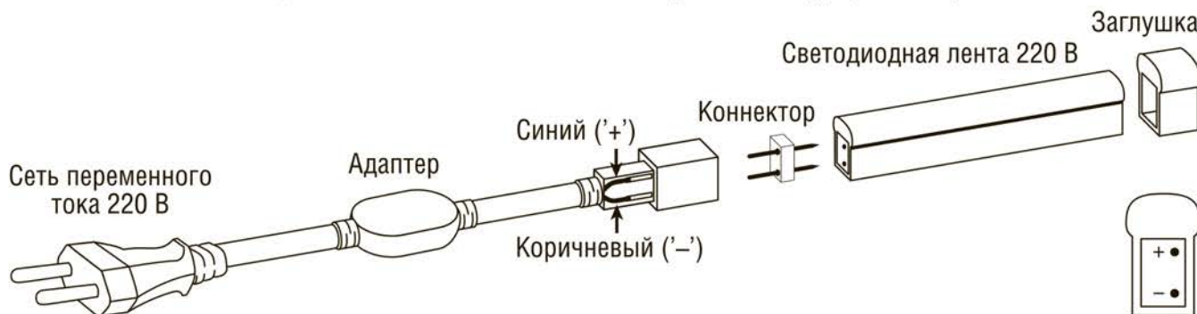
Рис. 1. Подключение светодиодной ленты 2835-220V-NEONLED.
