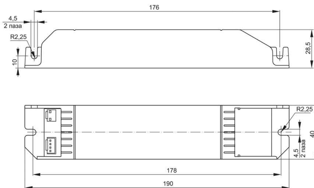
Рисунок 1 – Конвертер БАП40-1,0
