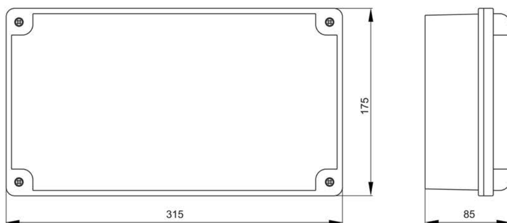
Рисунок 3 – БАП120-1,0, БАП200-1,0
