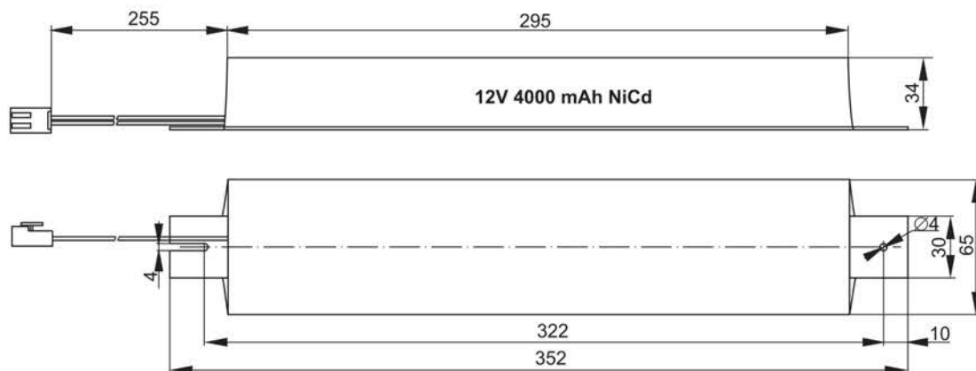
Рисунок 2 – Аккумуляторная батарея БАП40-1,0
