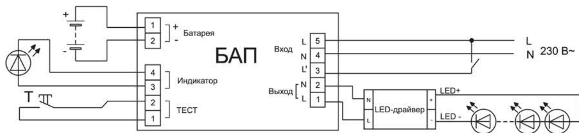
а) БАП40-1,0
