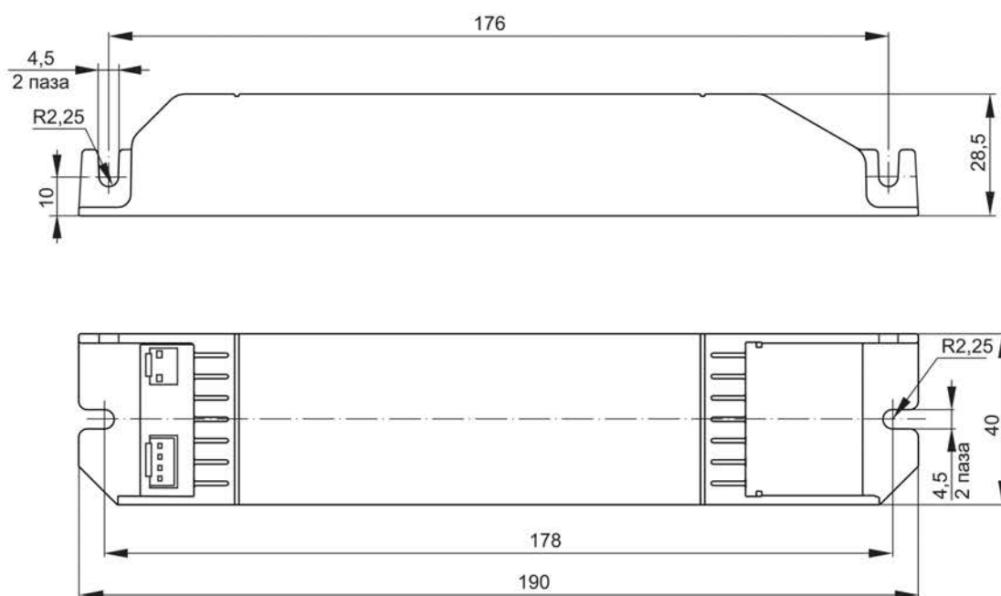
Рисунок 1 – Конвертер БАП40-1,0
