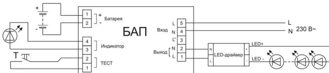
а) БАП40-1,0
