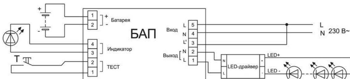
а) БАП40-1,0
