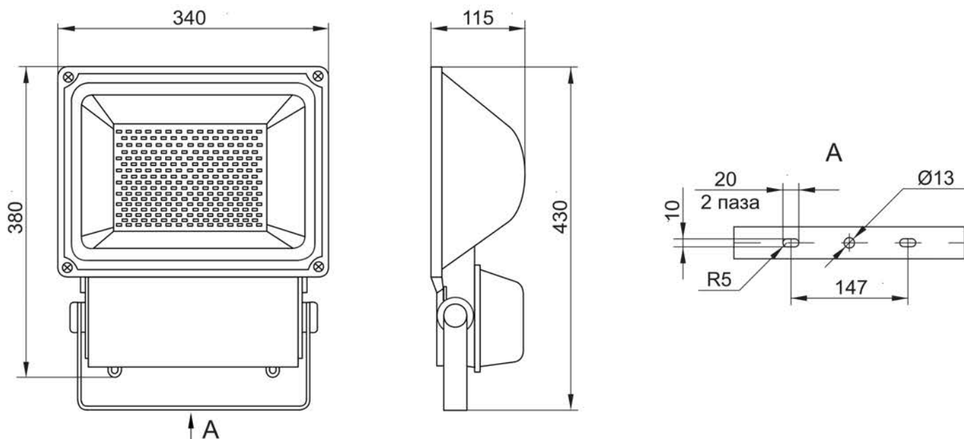
Рисунок 3 – Габаритные и установочные размеры прожектора СД004-200.
