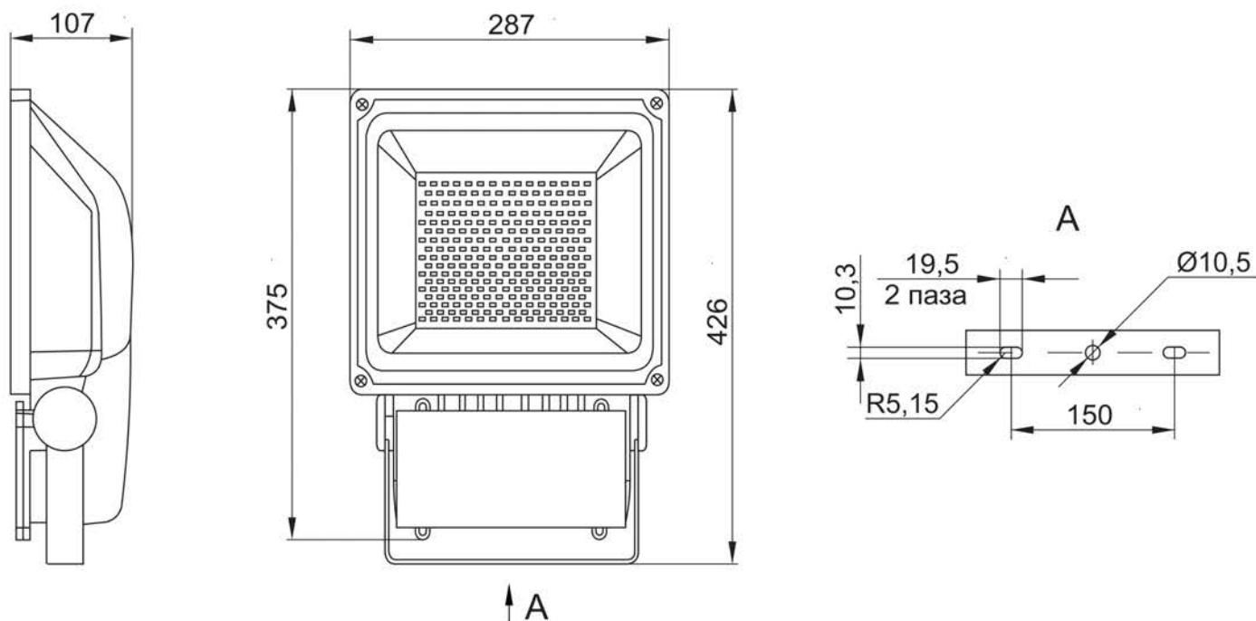
Рисунок 2 – Габаритные и установочные размеры прожектора СД004-150.
