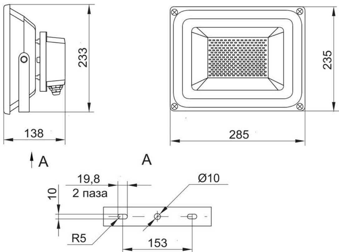
Рисунок 1 – Габаритные и установочные размеры прожектора СД004-100.
