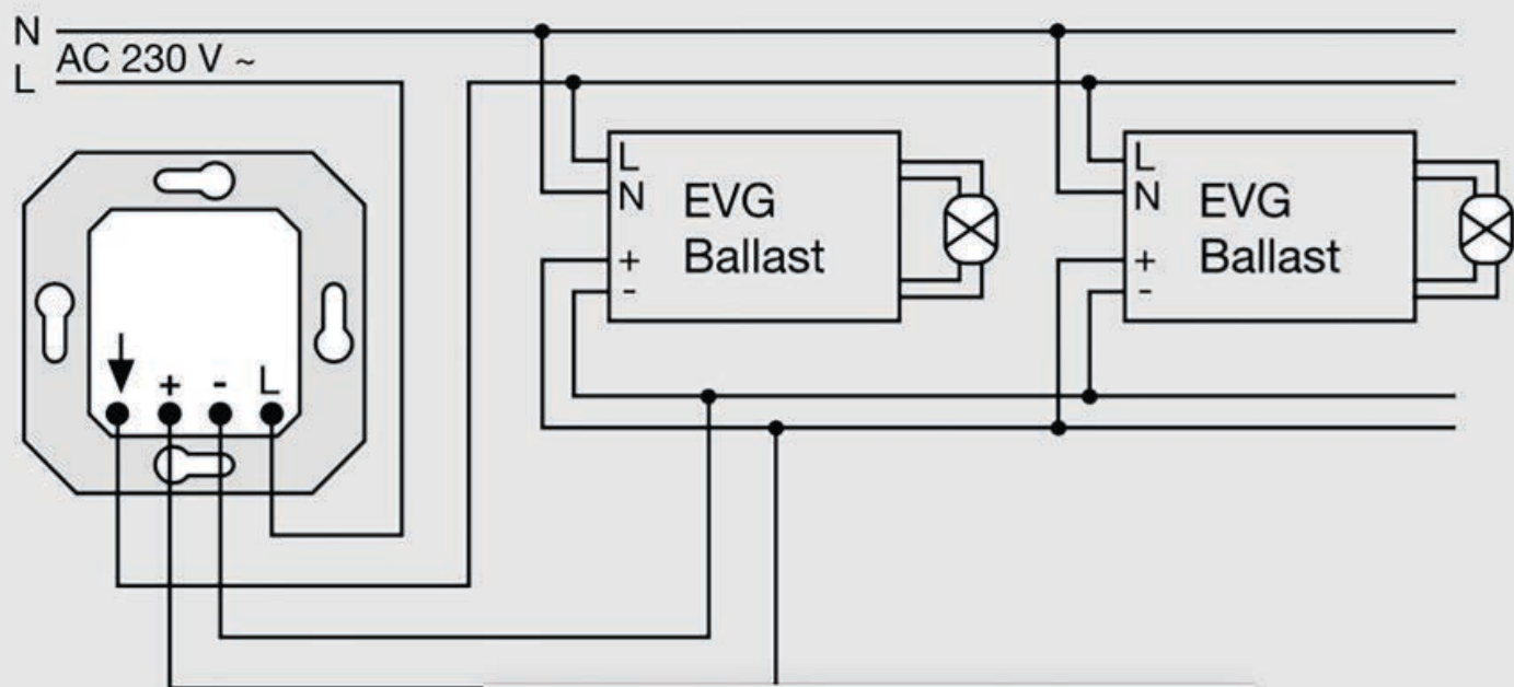
Схема подключения диммера 240-10 с дополнительным переключателем
