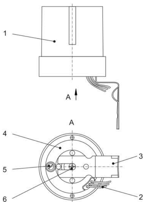
1 – защитный кожух; 2 – присоединительные провода (концы); 3 – крепёжный уголок; 4 – основание фотореле; 5 – регулятор уровня освещённости «LUX»; 6 – винт
