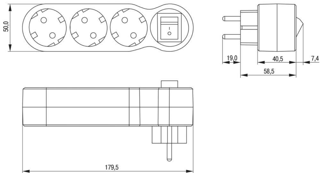
Рисунок 4 – Тройник Т-01/03В
