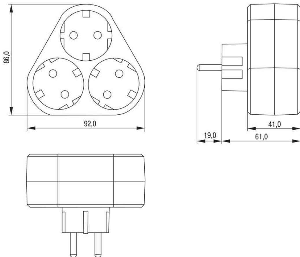
Рисунок 3 – Тройник Т-01/03
