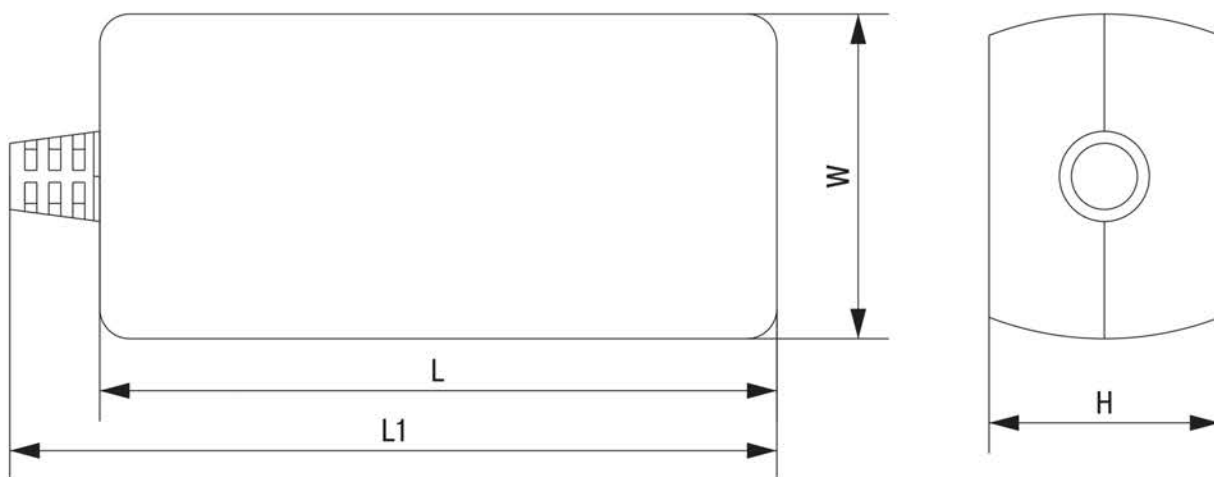
Рисунок 1 – Колодка удлинителя
