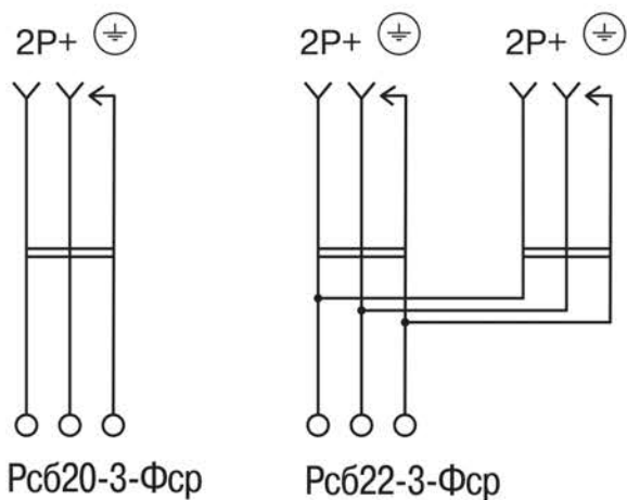
Рисунок 2 – Электрические схемы розеток серии «ФОРС»
