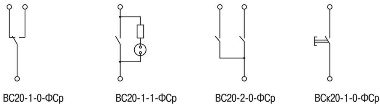
Рисунок 1 – Электрические схемы выключателей серии «ФОРС»
