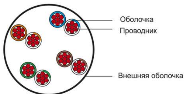
Рисунок 1 – Конструкция патч-корда категории 5е типа U/UTP
