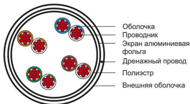
Рисунок 2 – Конструкция патч-корда категории 5е типа F/UTP
