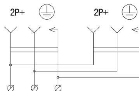
Рисунок 3 – Электрическая схема соединений РБ32-1-0м
