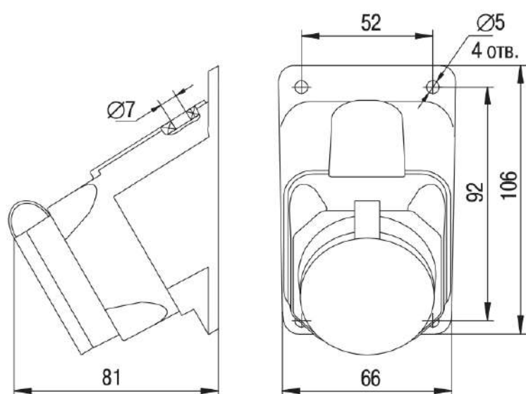
Рисунок 13 – Розетка с защитной крышкой угловая настенная РБy13-1-0м
