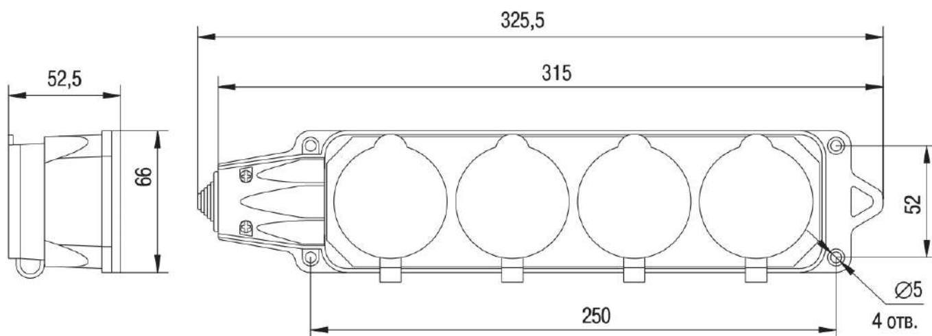
Рисунок 12 – Розетка (колодка) четырехместная с защитными крышками РБ34-1-0м
