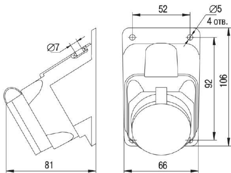
Рисунок 13 – Розетка с защитной крышкой угловая настенная РБ13-1-0м
