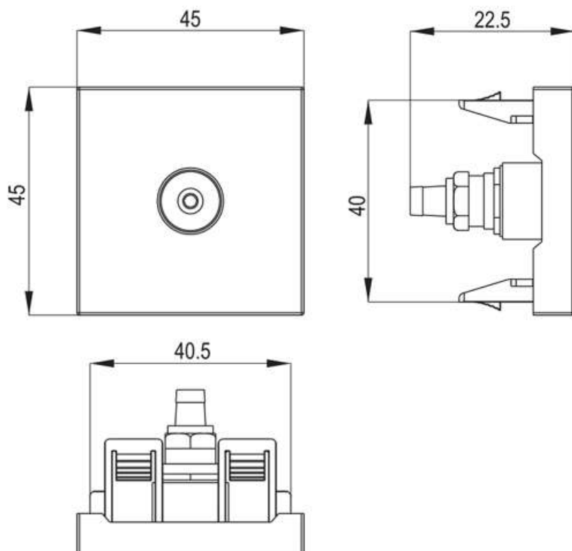
Рисунок 8 – Розетка телевизионная оконечная (на 2 модуля) РКТ-20-00-П
